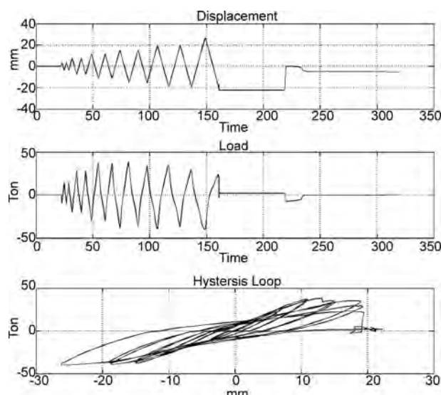
شکل ۱۴. منحنی اطلاعات خروجی جک.
