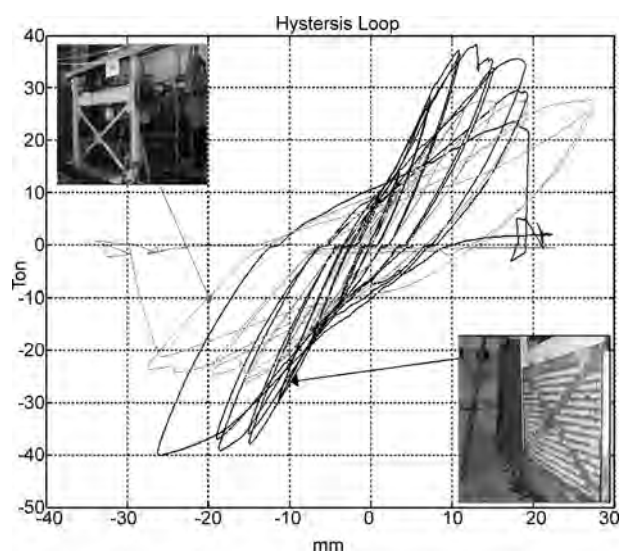
شکل ۱۶. منحنی هیستریزس دو آزمایش ۱- قاب فولادی با مهاربند ضربدری بدون میانقاب؛ ۲- قاب فولادی با مهاربند دارای میانقاب.
